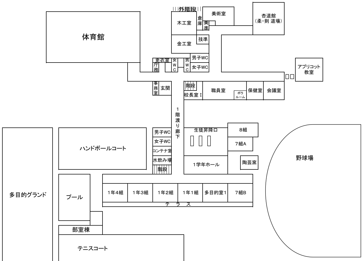
1階平面図
