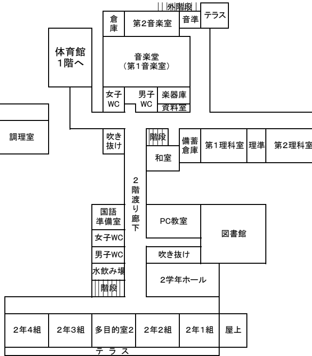
2階平面図
