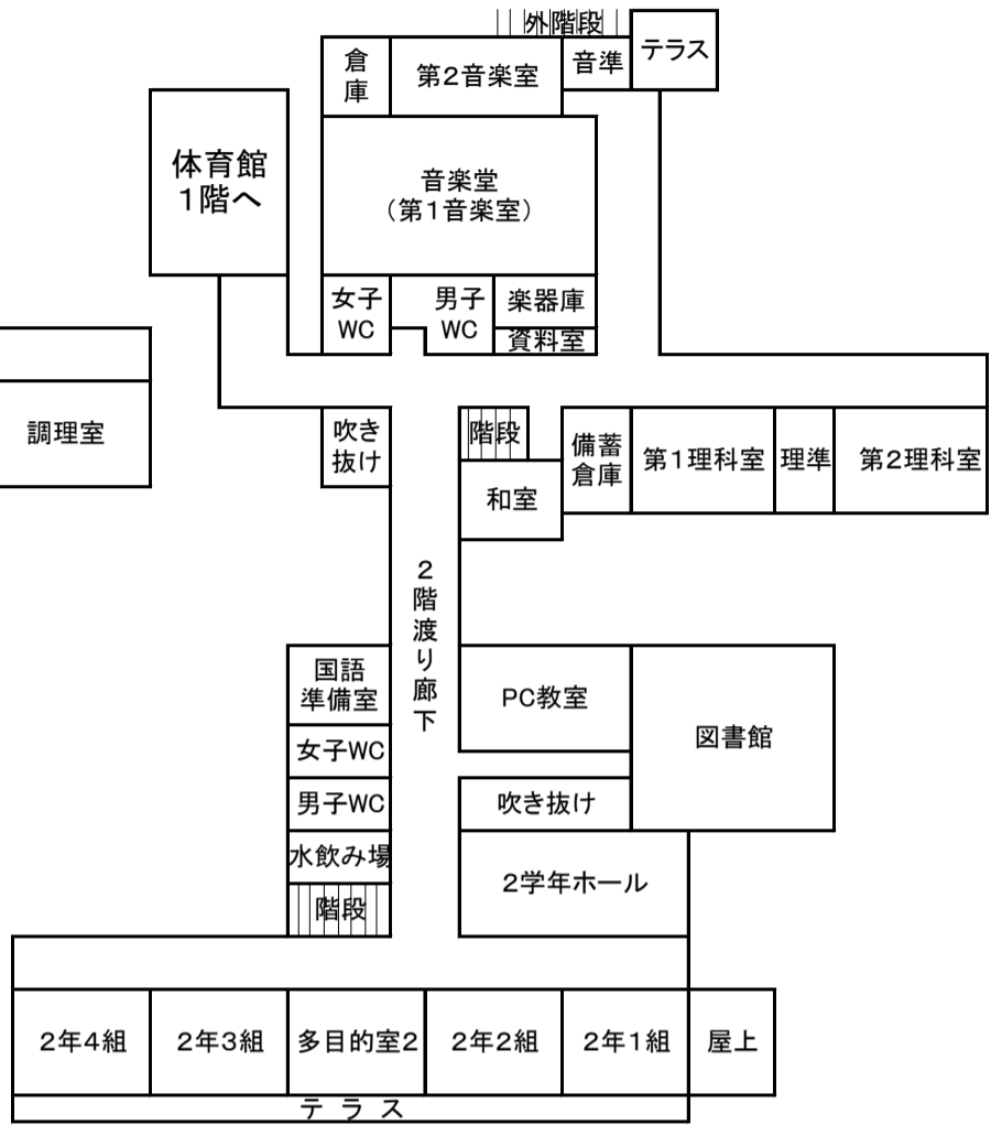
2階平面図
