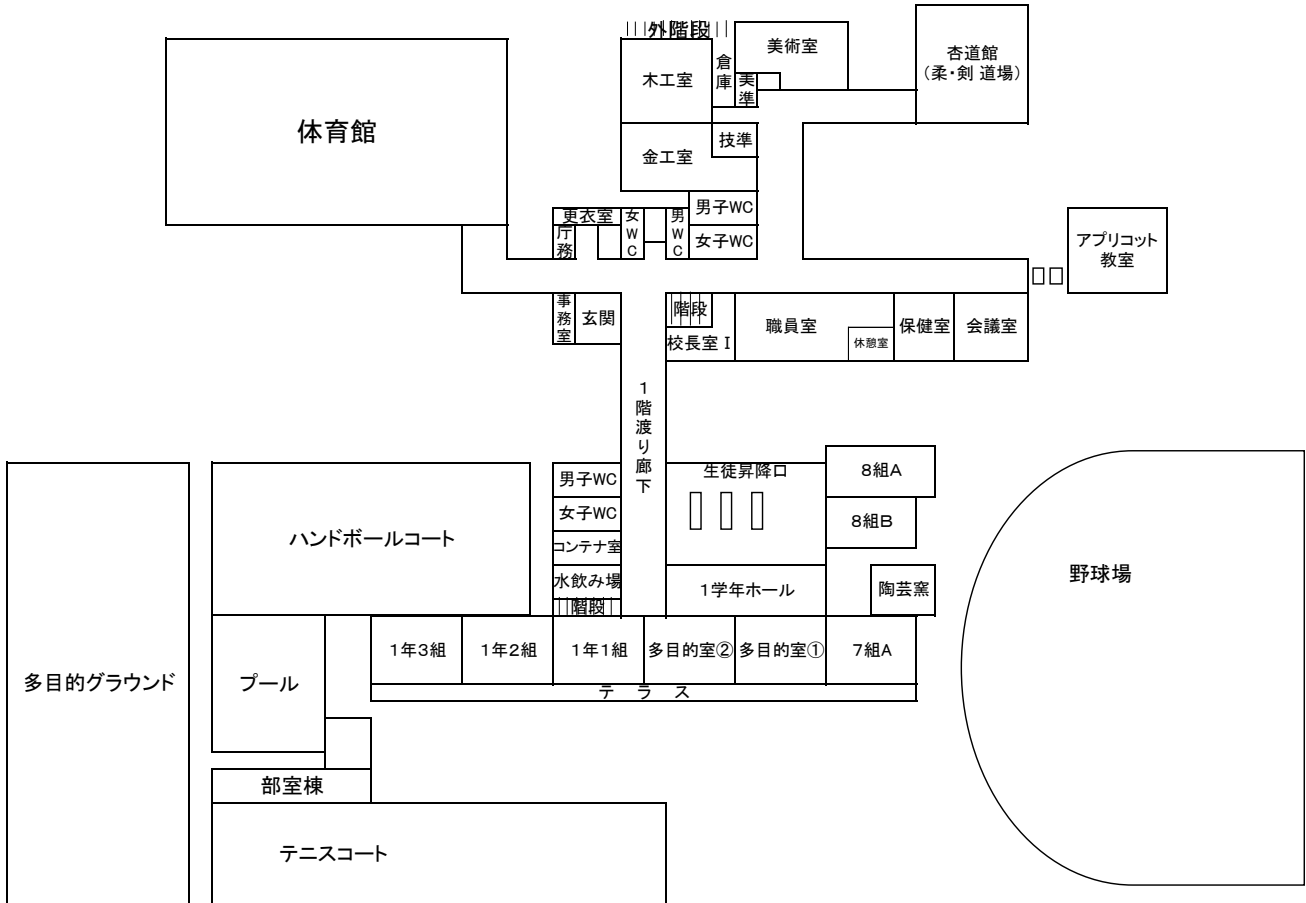
1階平面図
